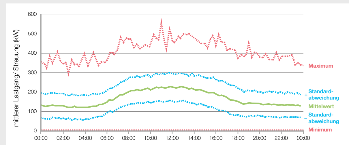
Lastgangverbrauch (Ø-Verbrauch an Werktagen) eines produzierenden Unternehmens
