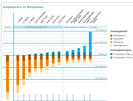
Abb. 1: Energiebedarf von Neubauten nach gesetzlichen Effizienzstandards 1977 bis 2009 Darstellung: www.co2online.de , 2015 Datenquelle: TU Darmstadt, Ergänzungen IFEU
