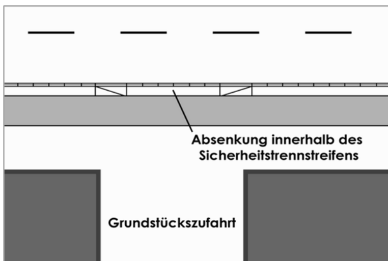
Abb. 28: Ausbildung einer Radwegüberfahrt mit Rampensteinen im Bereich von Grundstückszufahrten
