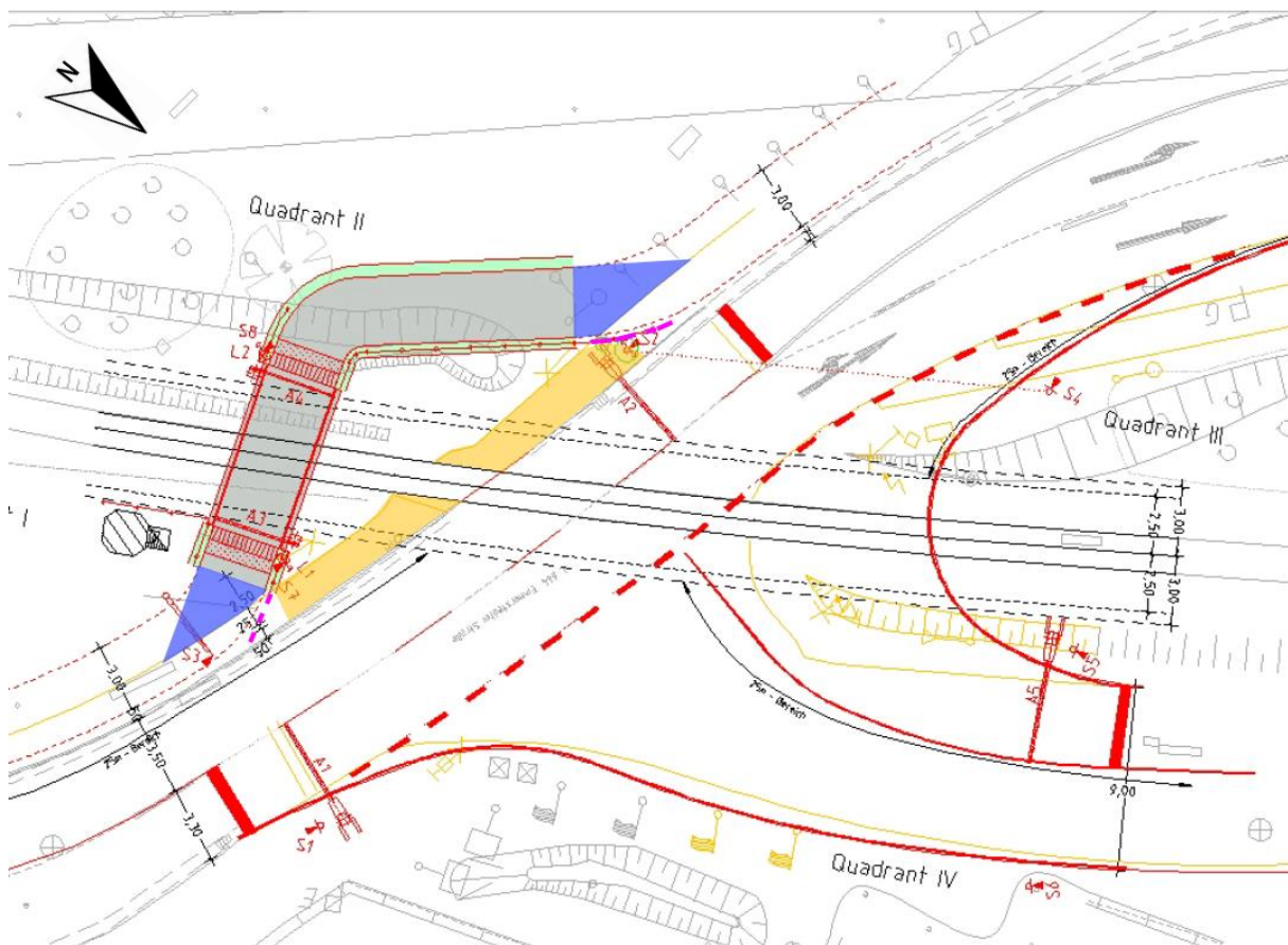
Abb. 25: Frühere Planung für den Ausbau des Bahnübergangs mit südlichem gem. Geh-/Radweg von 2017
