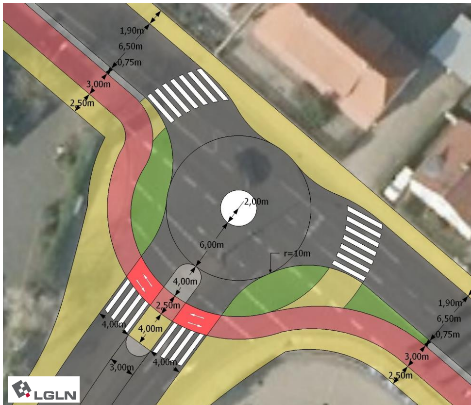
Abb. 32: Skizze Knotenpunkt Emmerstedter Str. / Industriestraße Variante A: Mini-Kreisverkehrsplatz (d=16 m) mit durchgehendem Zweirichtungsradweg
