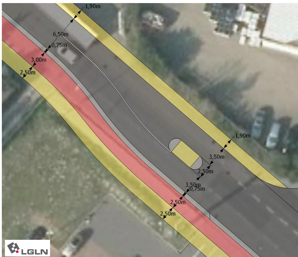
Abb. 29: Skizze Querungshilfe Variante A: Mit durchgehendem Zweirichtungsradweg und Grunderwerb
