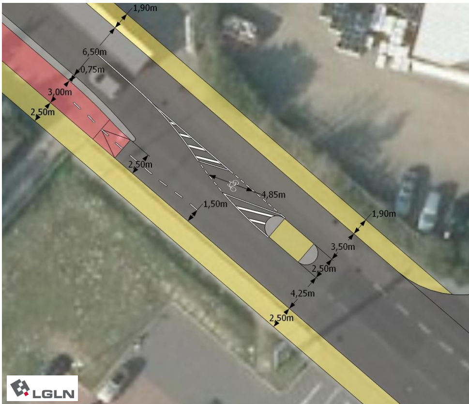
Abb. 31: Skizze Querungshilfe Variante C: Auflösung in gem. Geh-/Radweg mit separatem Radwegende und verkürzter Querungsdistanz am Radweganfang
