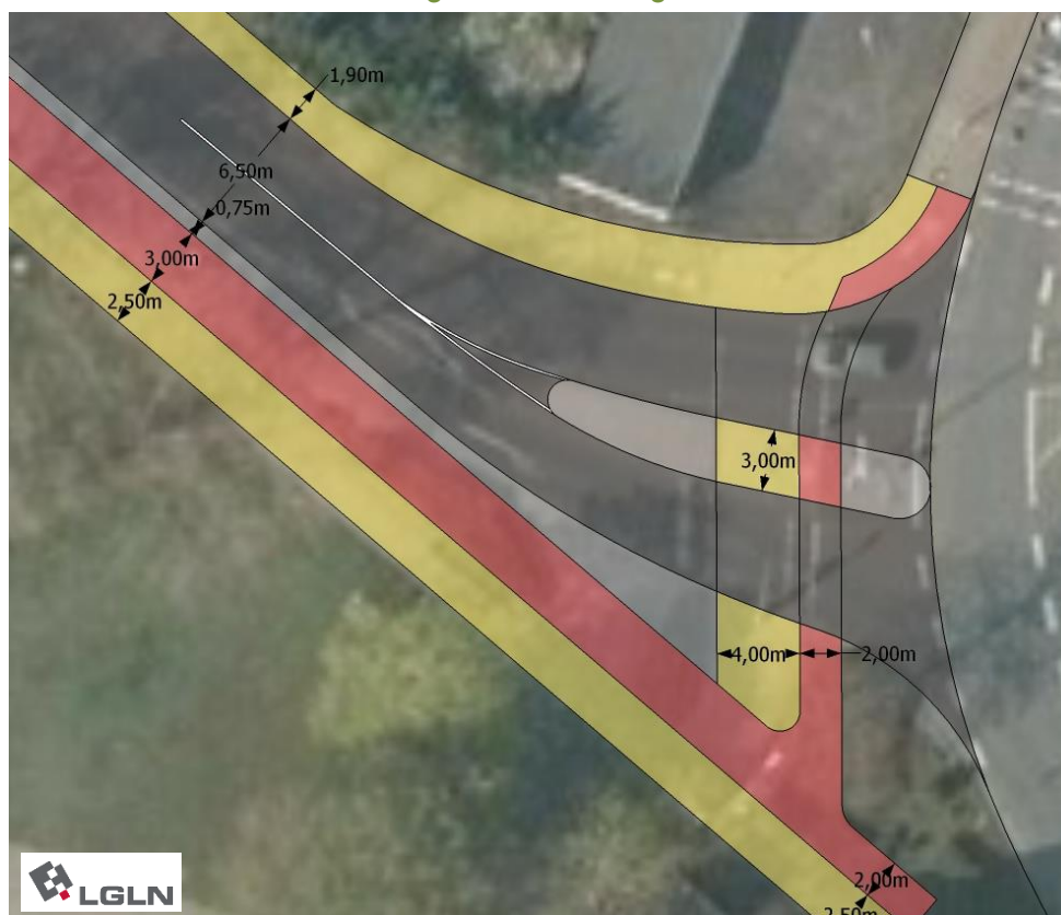
Abb. 34: Skizze Anschluss Knotenpunkt Konrad-Adenauer-Platz Variante A: Anschluss eines durchgehenden Radweges auf der Südwestseite
