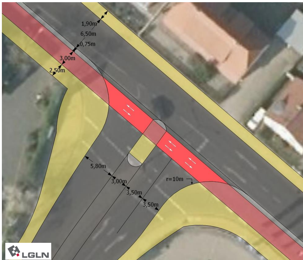
Abb. 33: Skizze Knotenpunkt Emmerstedter Straße / Industriestraße Variante B: Einmündung mit Radfurt für den durchgehenden Zweirichtungsradweg
