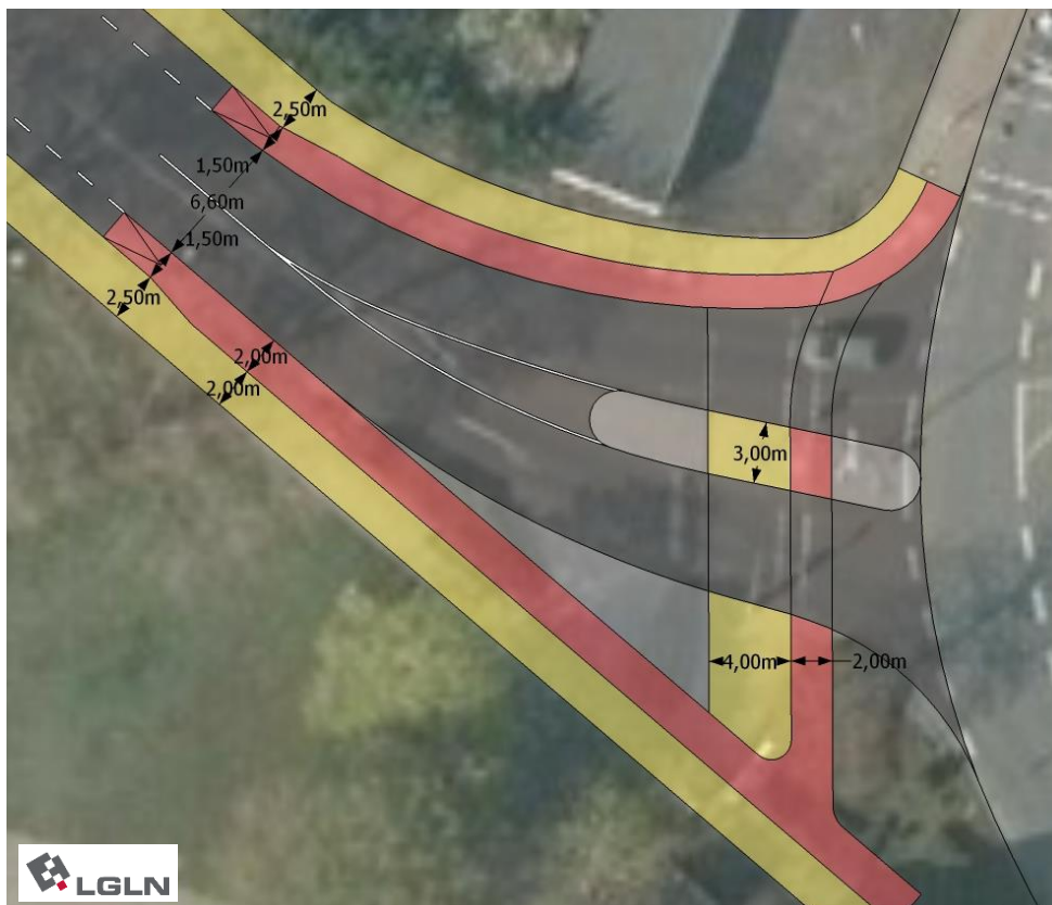
Abb. 35 Skizze Anschluss Knotenpunkt Konrad-Adenauer-Platz Variante B: Führungswechsel Fahr- bahn / Radwege im Seitenraum mit sicherem Radwegende
