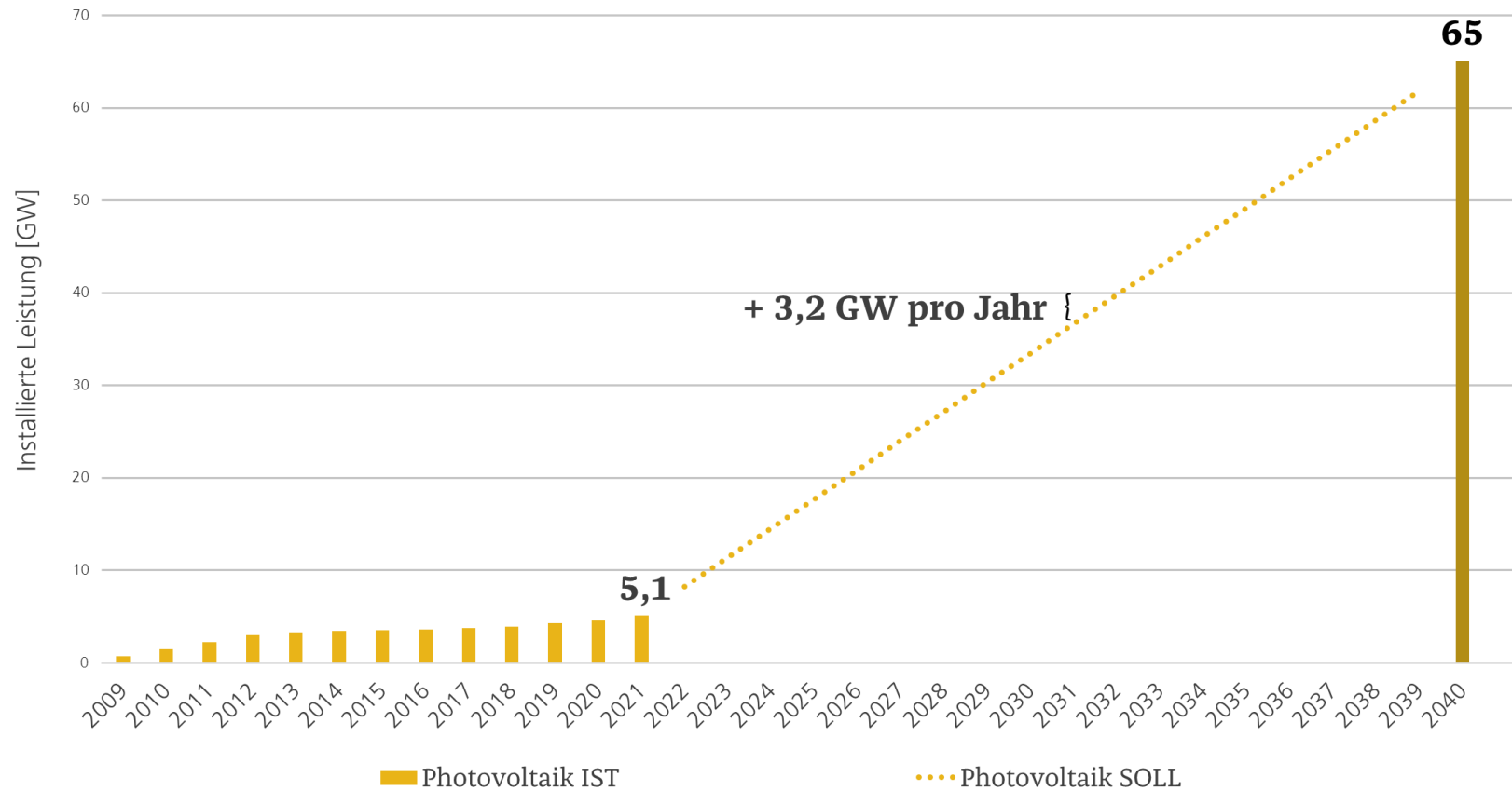
Installierte Leistung Photovoltaik in Niedersachsen mit Ausbausziel 65 GW in 2040
